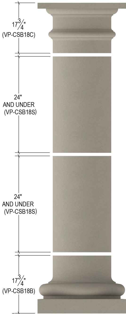
VP-CSB18
