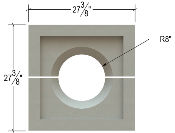
VP-CSB18C
